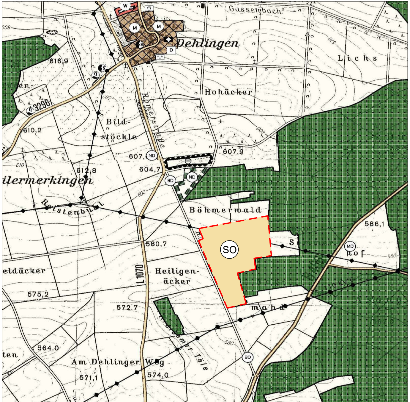
Planzeichnung M 1:5000
